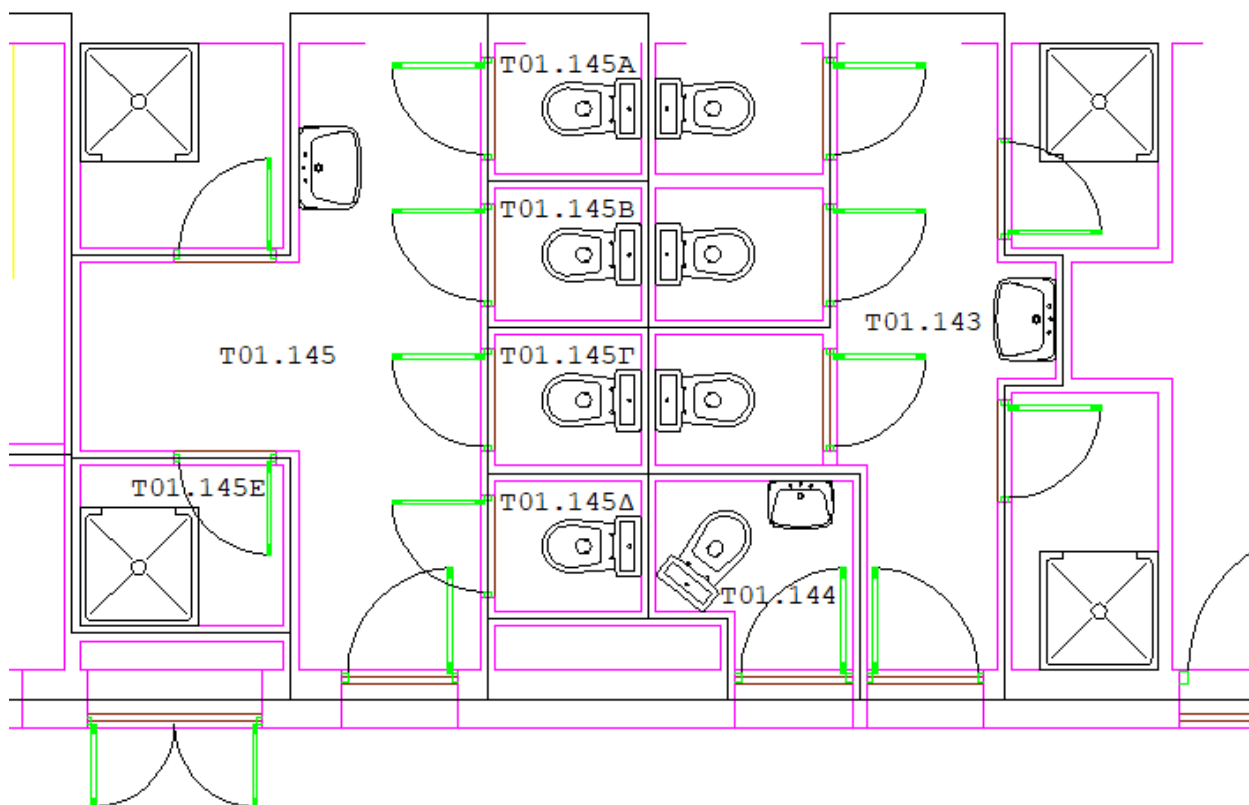
Σκαρίφημα 1 (1ος όροφος κτιρίου Α πτέρυγας Τσαγκάρη)
